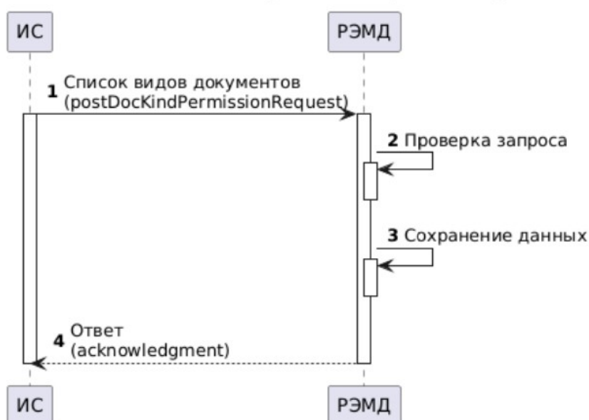
Рисунок 6 – Сценарий передачи списка соответствий "МО – виды документов"
