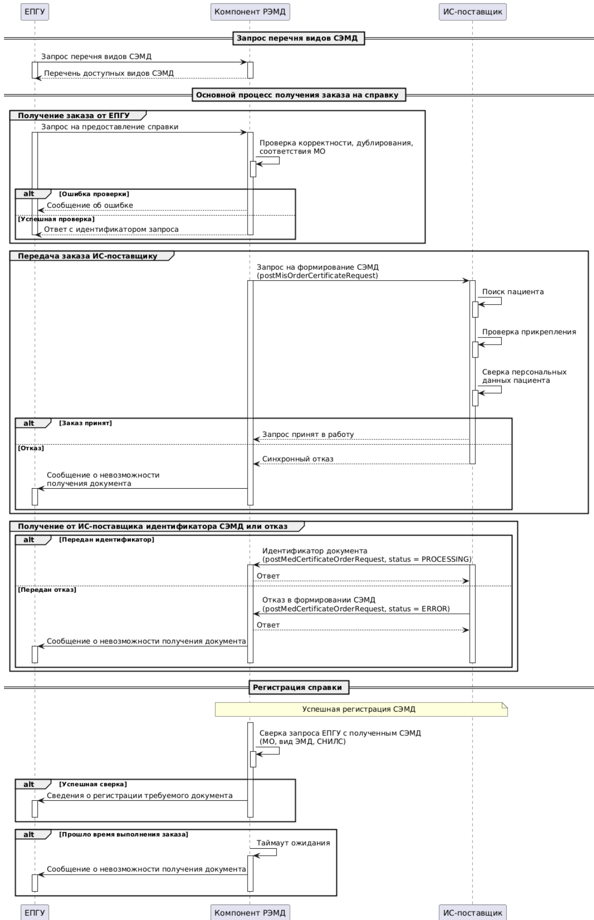
Рисунок 7 – Сценарий предоставления услуги в рамках сервиса "Заказ справок онлайн"
